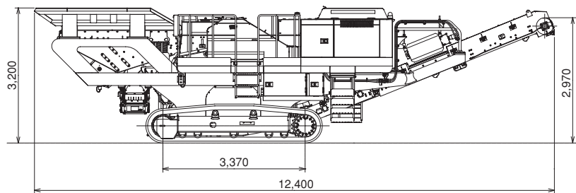
BR380JG-1 (稼働時) (単位：mm)
