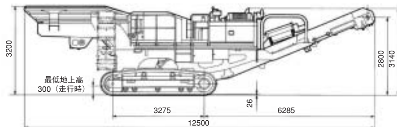
BR380JG-1 (稼働時) (単位：mm)
