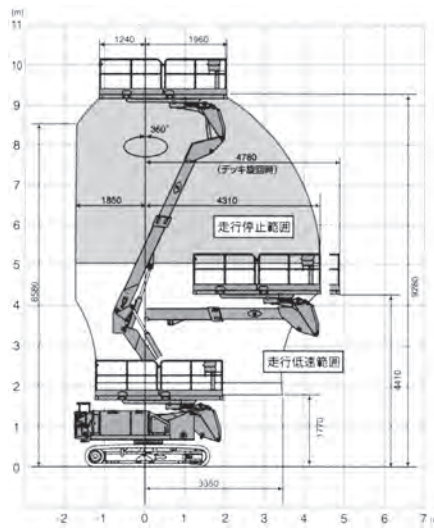
■作業範囲図(単位:m)
