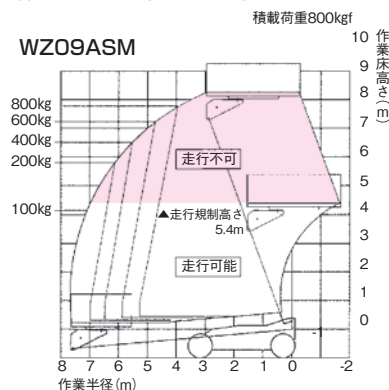
■作業範囲図(単位:m)
