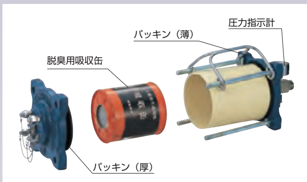
エアラインマスク AL-4N
