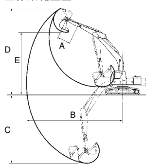
■標準アームおよびエクステンションアーム使用時の作業範囲表（バックホー）
