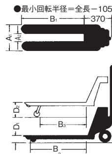
■寸法図 (単位: mm)
