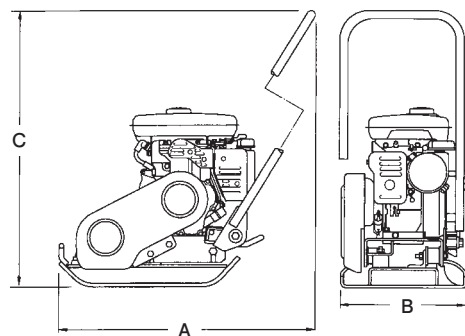
■寸法図(単位: mm)
