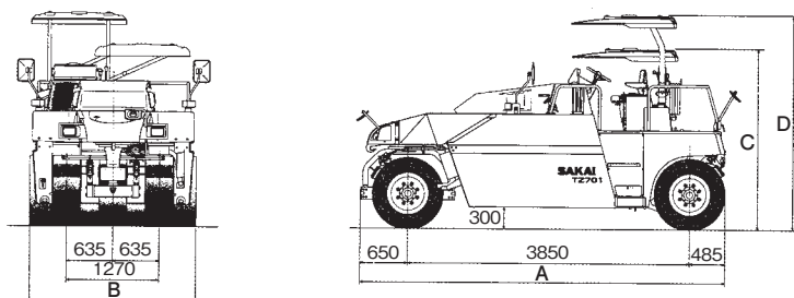
TZ701 ■寸法図(単位: mm)
