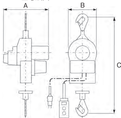
■寸法図
